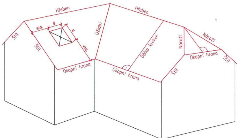
Obrázek 1: Schéma rozměření střechy pro vyhotovení kladečského plánu
